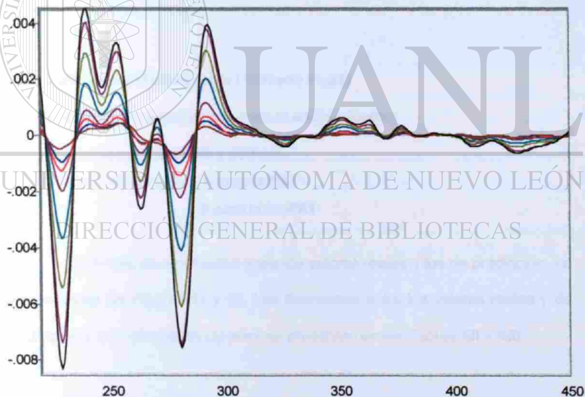
Figura 12 Espectros de absorción de IsoPA1 en 2ª derivada Concentraciones de 0.8 a 10 µg/mL
