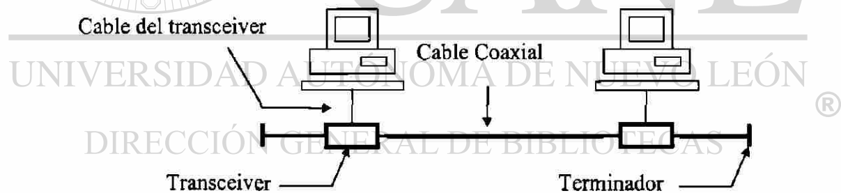
Figura 3-5 Componentes de una red Thick Ethernet
