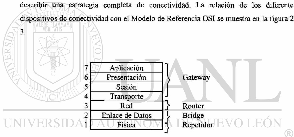
Figura 2-3 Dispositivos de Conectividad y el Modelo de Referencia OSI.
