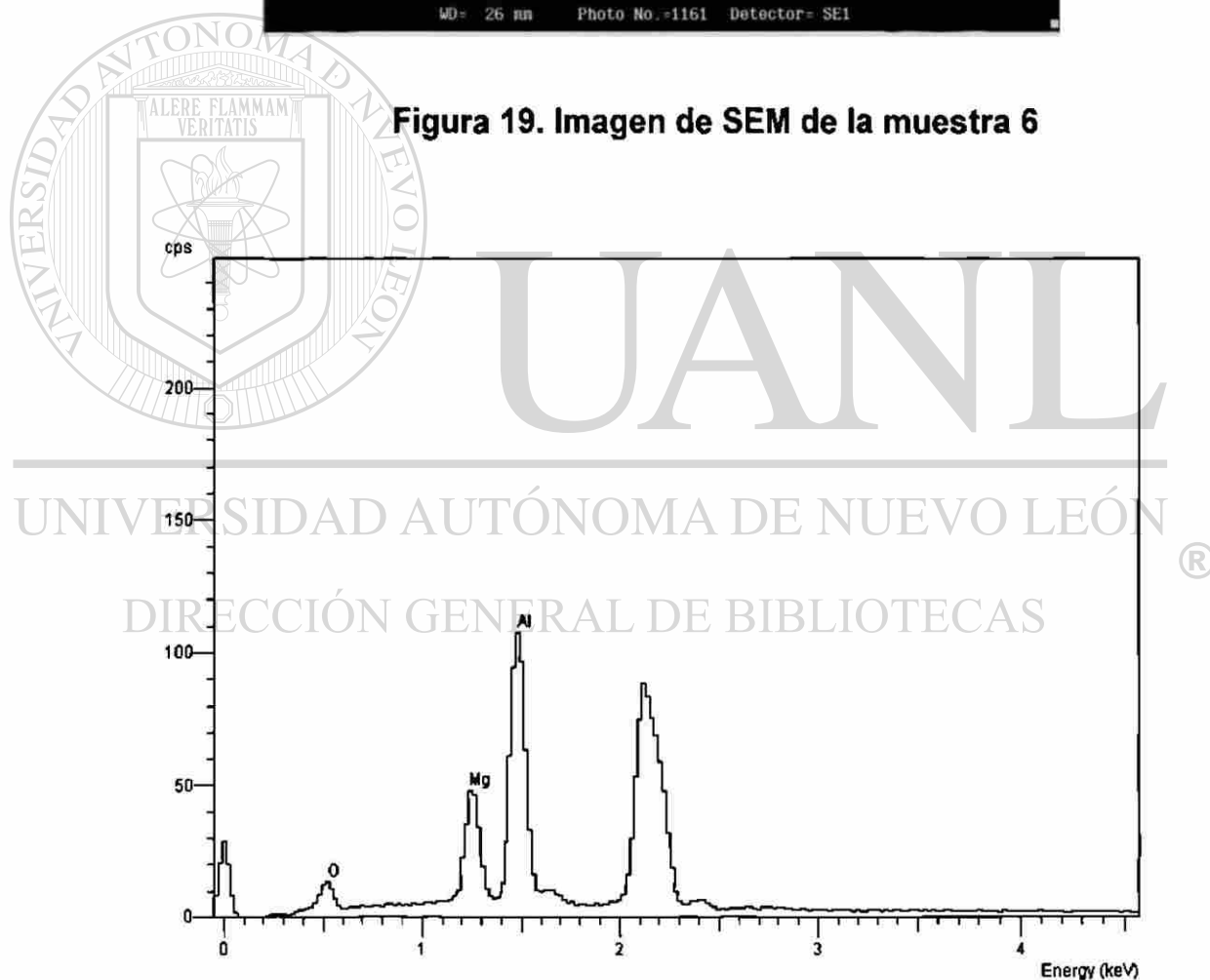
Figura 19 (a). Espectro correspondiente al análisis realizado a la región 6 de la muestra 6.
