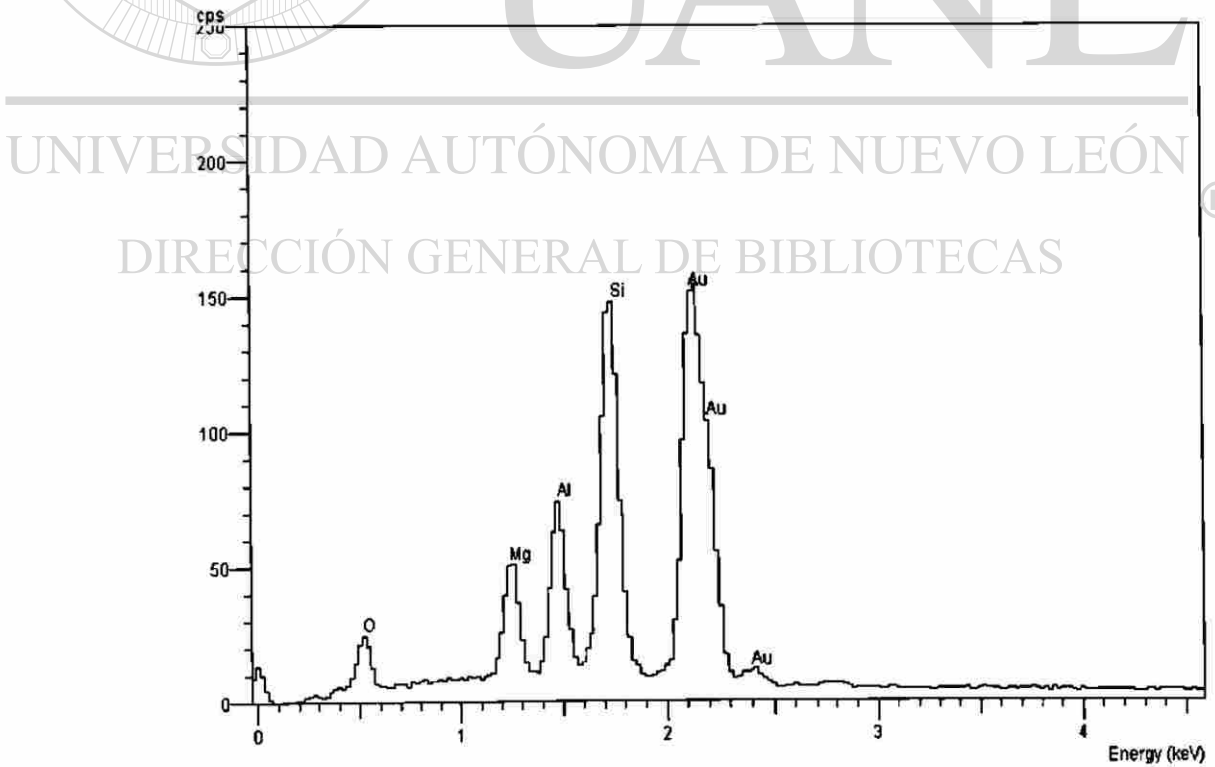
Figura 18(a). Espectro de la región 4 de la imagen de SEM 1.
