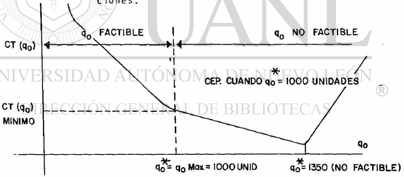
Gráfica 6.1. Cantidad económica de pedido con restricciones.
