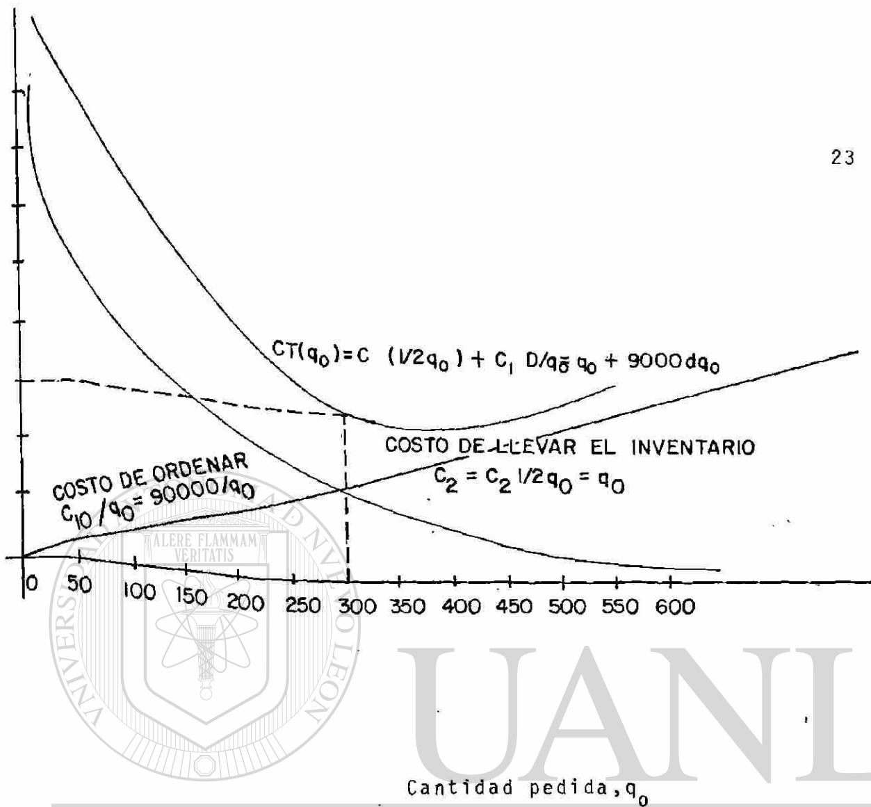
Figura 5.3. Curvas de costo del modelo clásico CEP; donde la D = 1000 unidades X año, C_2 = \$2.00 por unidad por año, C_1 = \$9.00 por orden
