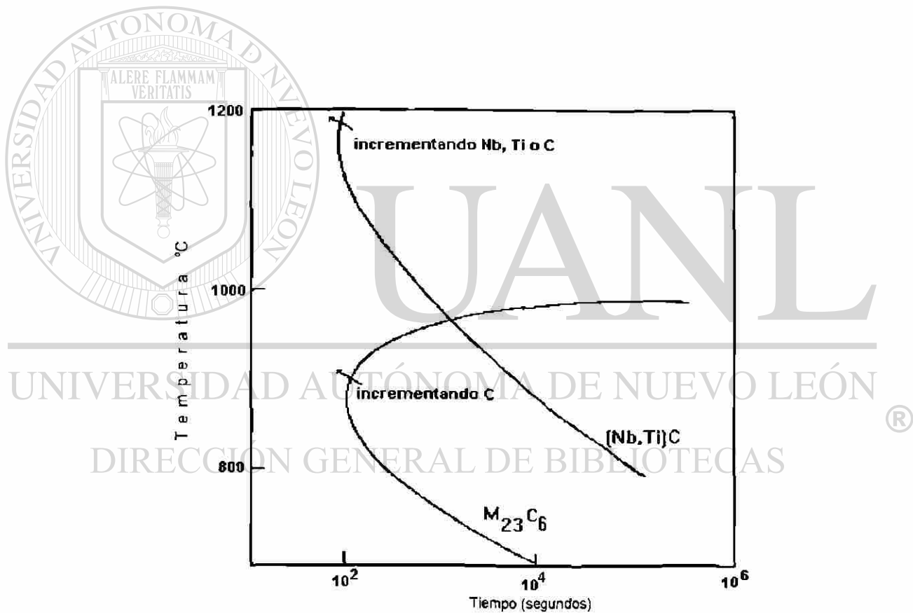
Figura 3.18 Crecimiento de la curva TTP para carburos de cromo ( M_{23}C_6 ) y Nb(Ti)C en aceros inoxidables Cr-Ni [11].
