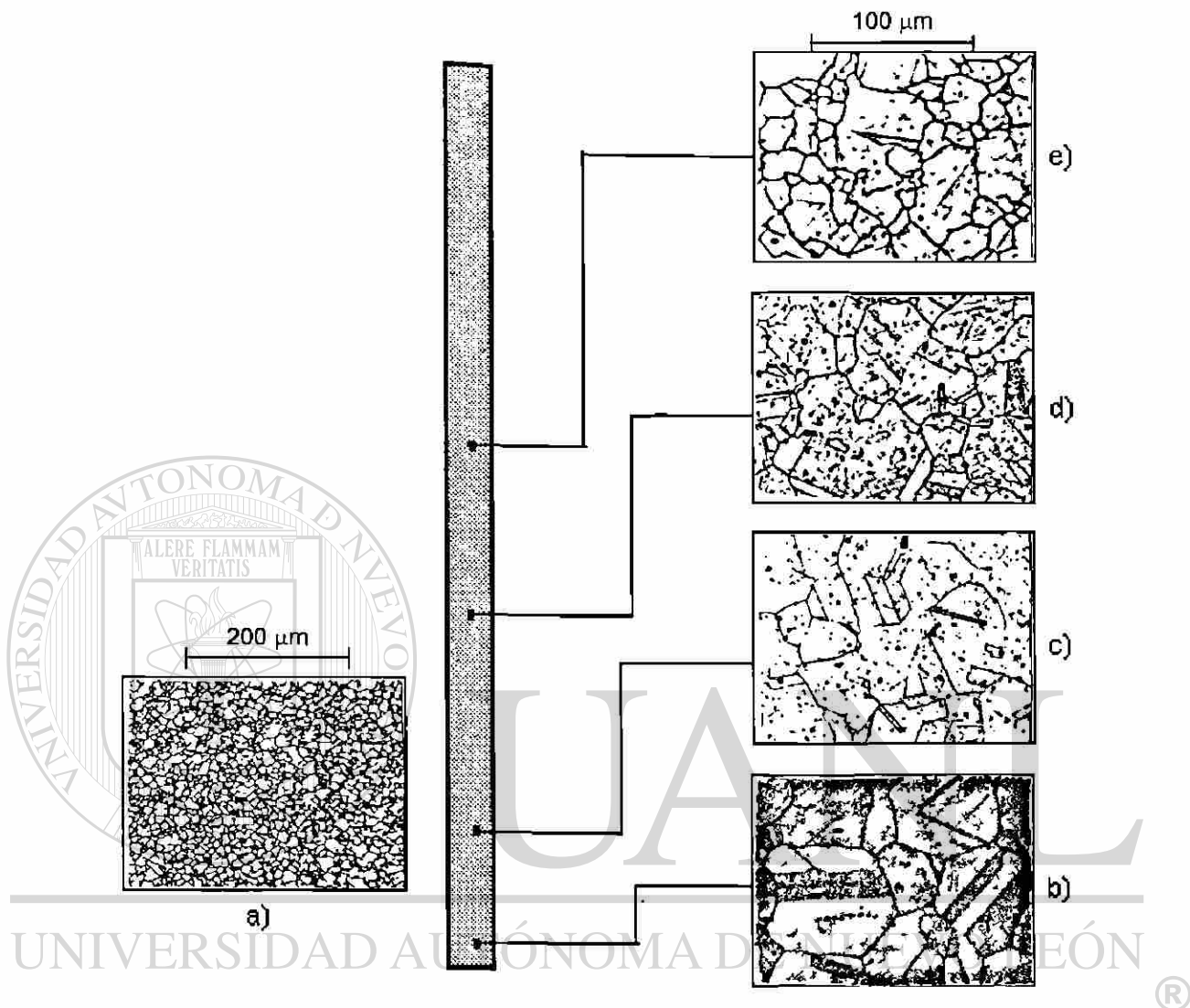
Figura 5.4 Metalografías obtenidas de una barra de acero inoxidable y atacada electroquímicamente ( \text{HNO}_3 al 93 % y 1.1 VCD). a) Sin tratamiento térmico, b) a e) enfriada en agua a través de uno de sus extremos a 0.5, 4, 8, 16 cm de dicho extremo respectivamente.
