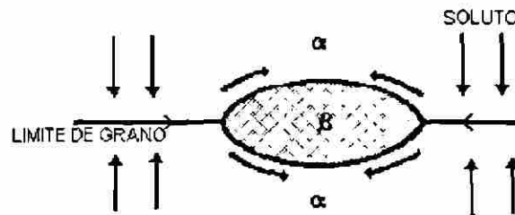
Figura 3.13 La difusión en el límite de grano ocasiona un rápido alargamiento y crecimiento de precipitados limítrofes [17].
