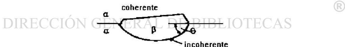
Figura. 3.8 El tamaño del núcleo crítico puede ser reducido formando una interfase coherente de baja energía con uno de los granos [17].
