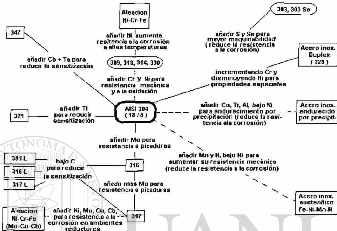
Figura 2.6 Modificaciones a la composición del acero AISI-304 para la obtención de propiedades especiales. Las líneas interrumpidas representan líneas composicionales hacia otros sistemas de aleaciones [2].
