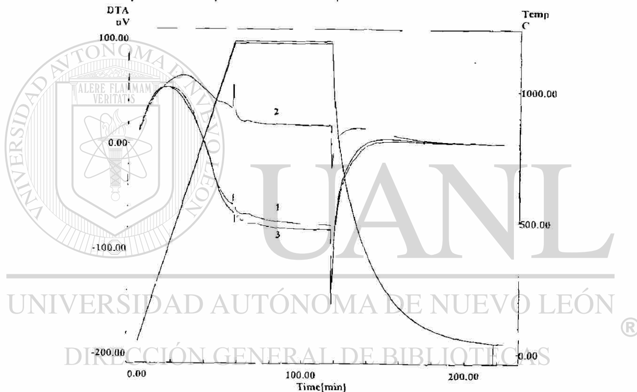
Figura 5.11 Ciclo térmico para muestras de acero inoxidable con diferente tratamiento térmico experimentadas en el DTA. 1. Sin tratamiento térmico, 2. porción enfriada rápidamente, 3. porción enfriada lentamente.
