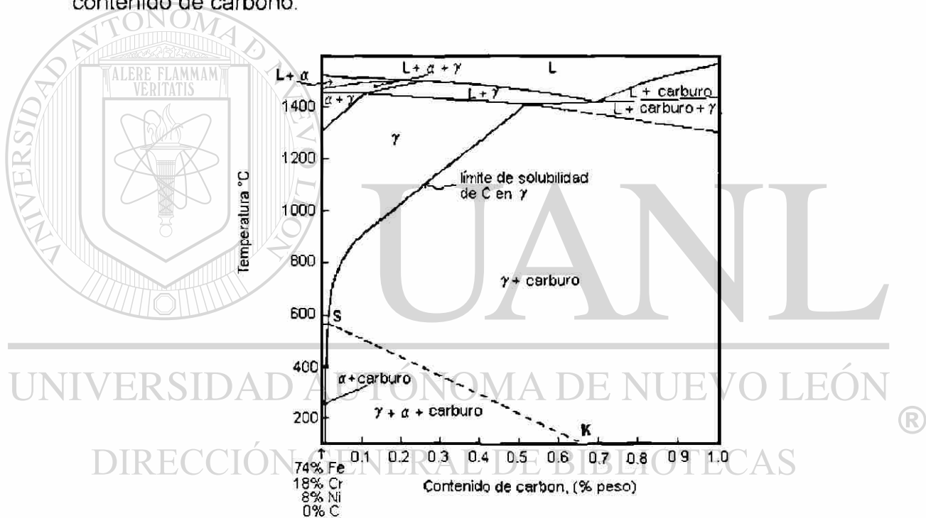
Figura 3.16 Efecto del carbono en un diagrama de fases del acero AISI 304 (18% Cr, 8% Ni) [2].
