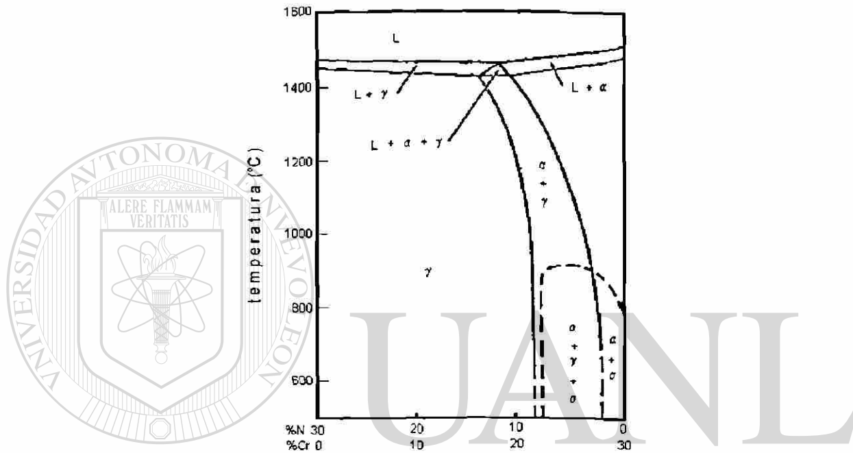
FIGURA 2.3. Sección vertical del diagrama de fases Fe-Cr-Ni a 70 % en peso de Fe [19]
