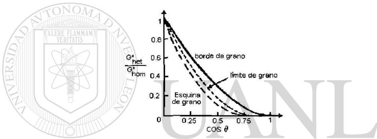
Figura 3.7 Efecto del ángulo \theta en la energía de activación para límite, borde y esquina de grano [17].
