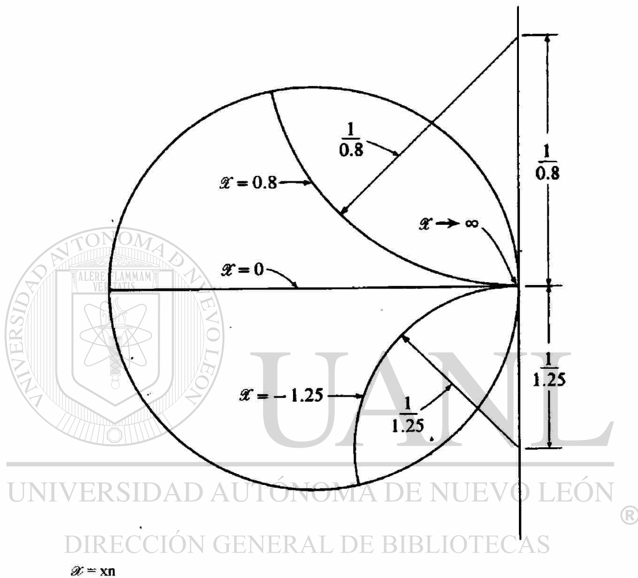
Figura iv-3.- Lugar geométrico de la reactancia
