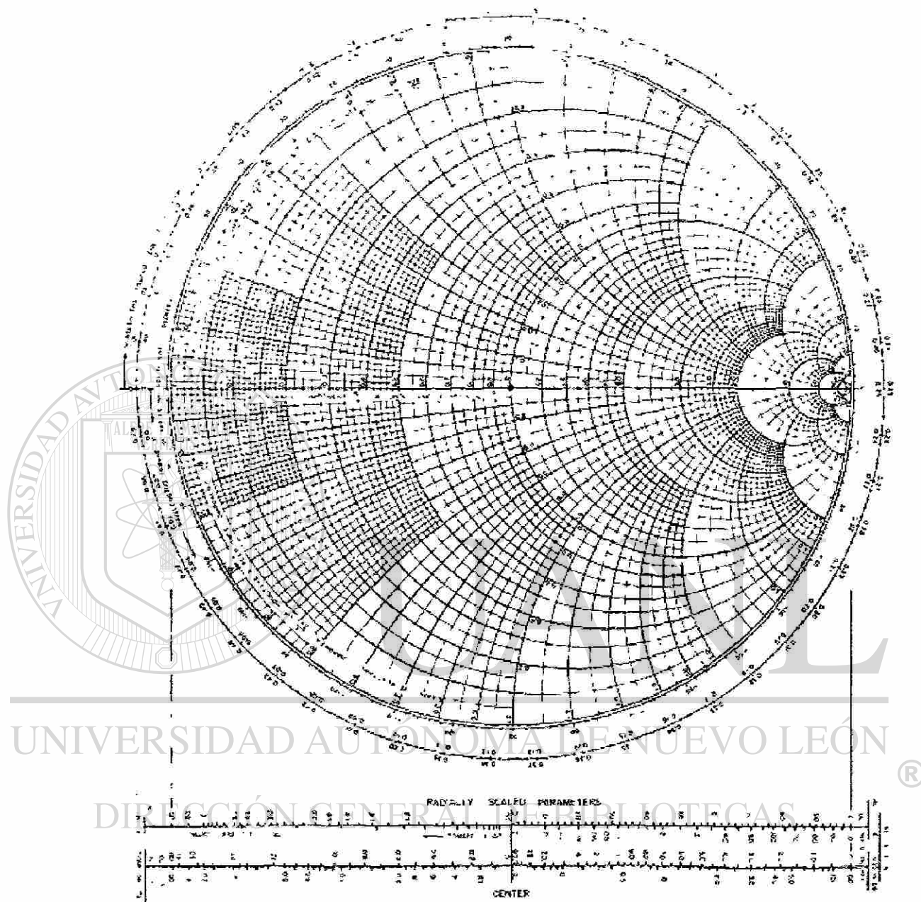
Figura iv-4.- Carta de Smith
