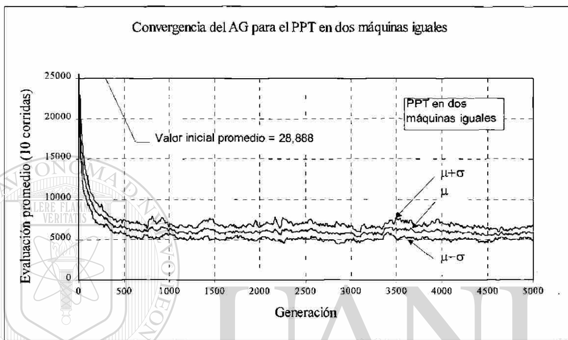
Figura 5.4. Convergencia del AG para el PPT en dos máquinas iguales con 50 tareas incluyendo costos de preparación.
