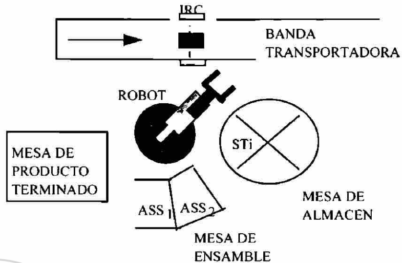
Figura 2.2. Célula de Ensamble
