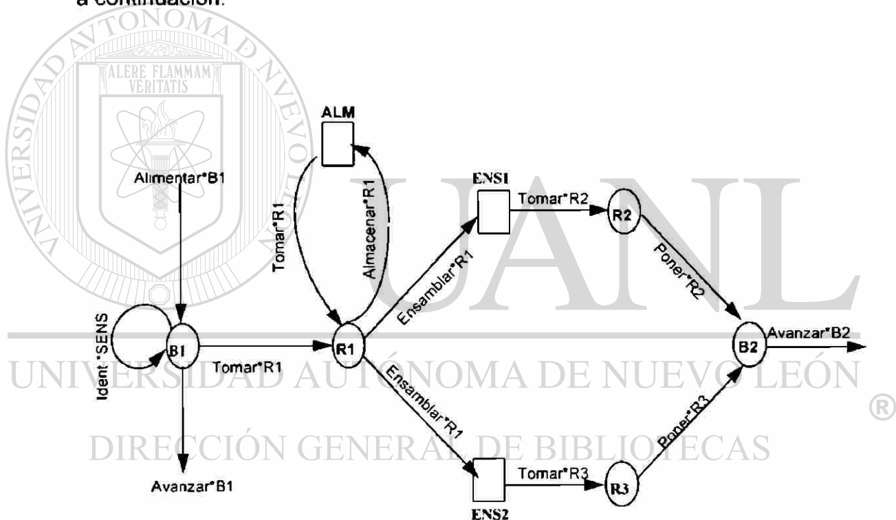
Figura 6.3 Grafo de la célula de ensamble del ejemplo 1
