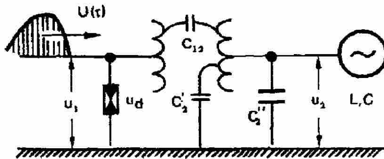
Protección de un transformador de potencia trifásico (Del-Est), el cual opera en bloque con un generador (las capacitancias son hipotéticas)
