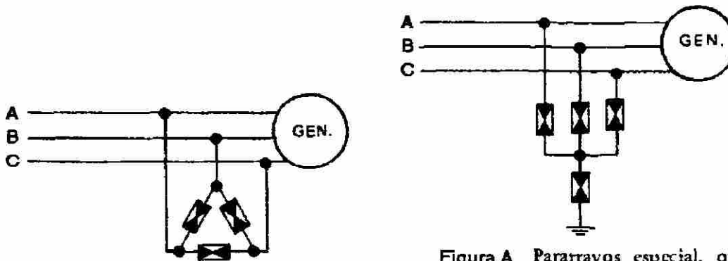
Figura A Pararrayos especial, que combina las funciones de los seis (6) anteriores y de diseño convencional, con un sustancial ahorro de dinero y espacio. Los cuatro pararrayos señalados forman una sola pieza.
