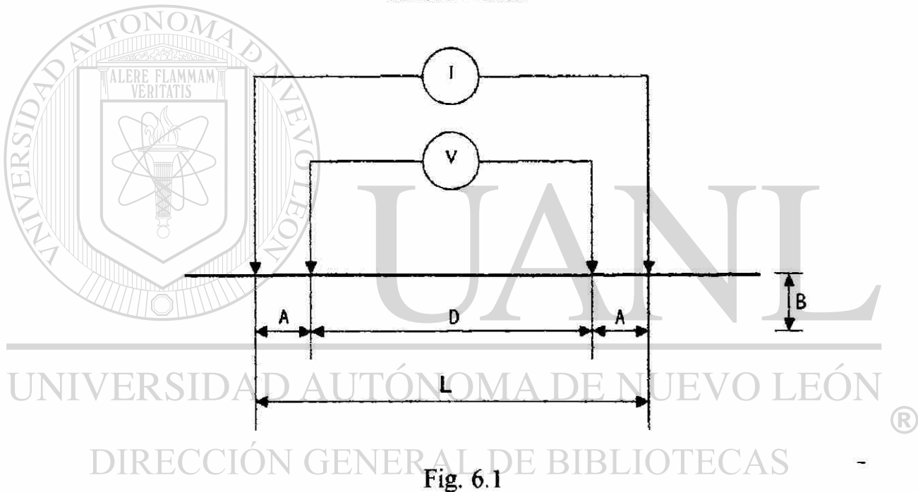
Método Wenner
