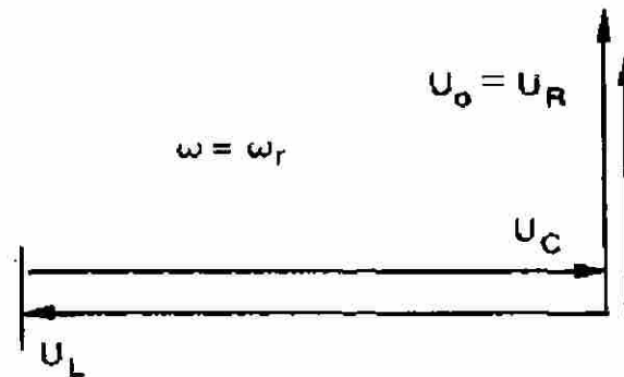
Circuito en resonancia
