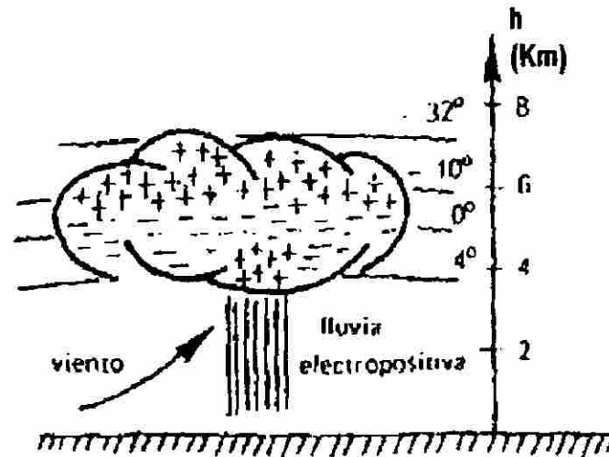
Nube según Simpson Con alturas e isotermas más usuales
