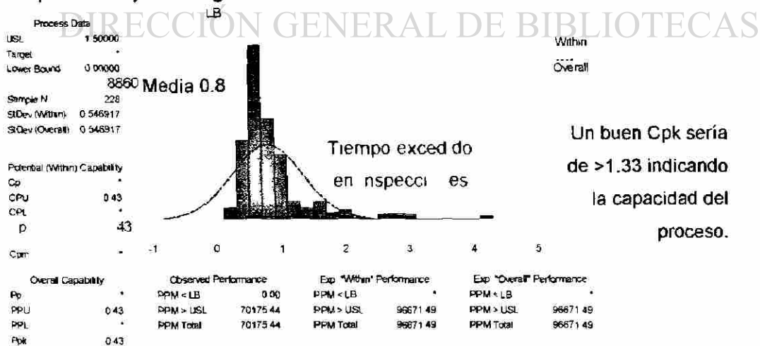
Fig. 14 Histograma de la Capacidad del proceso
