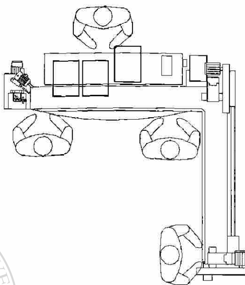
Figura 10.1.2 Otro tipo de arquitectura de línea o celda de manufactura teniendo en forma de "L" ó "U". Este tipo de arquitectura son muy usados en las fabricas donde se utiliza una manufactura flexible, ya que la ventaja de estas lineas es que son diseñadas para fabricar productos estando las 4 personas presentes o solo dos dependiendo el volumen requerido.
