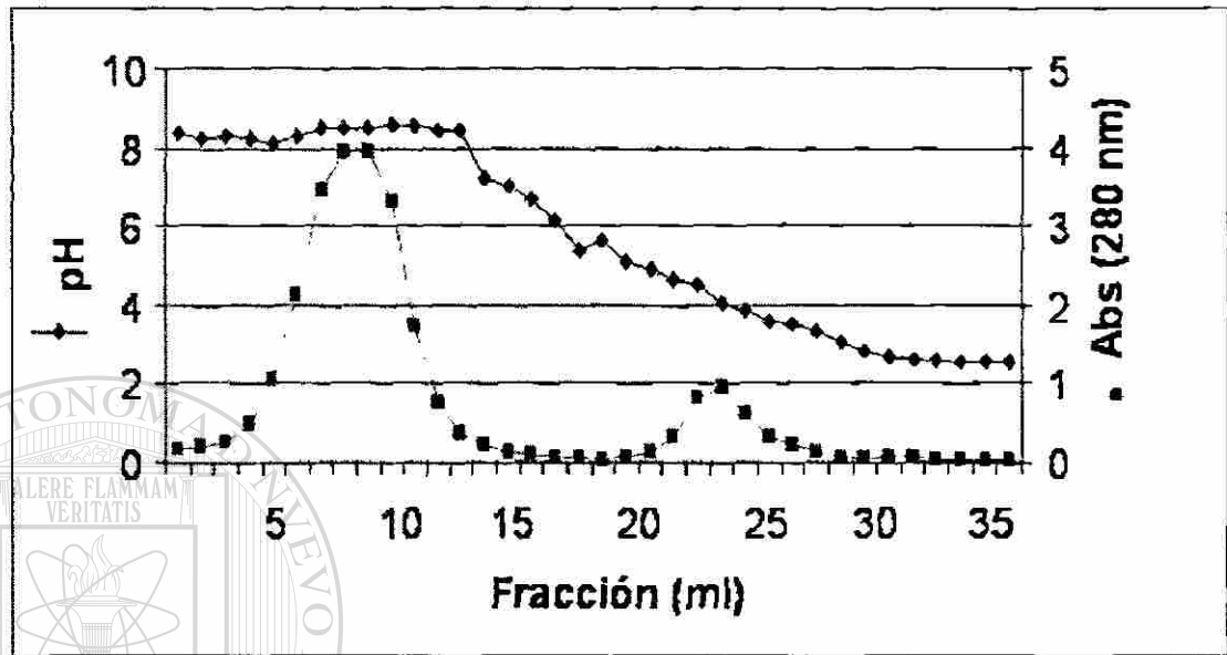
Figura 15. Espectro de elución de los IgG (fracciones 5 a 10) separados con Proteína A.
