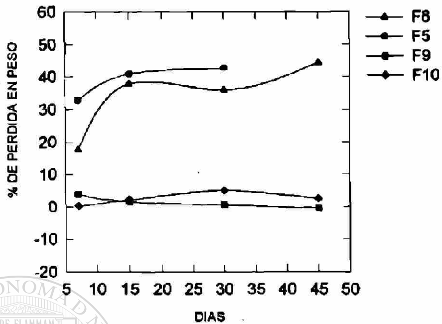
Fig. 1 Porcentaje de pérdida en peso en membranas del grupo 4 expuestas al consorcio LD-76 en laboratorio por 45 días.
