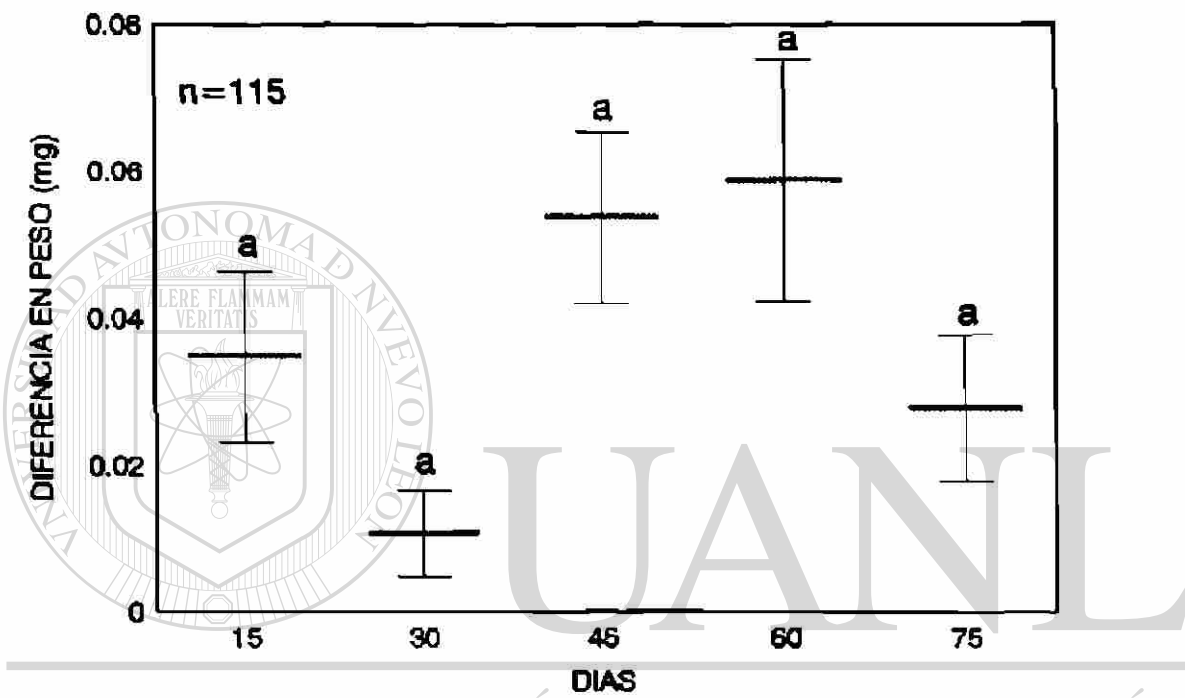
Fig. 10 Diferencia de Peso en las fechas de colecta del experimento en laboratorio con Serratia marcescens en los diferentes formulados.
