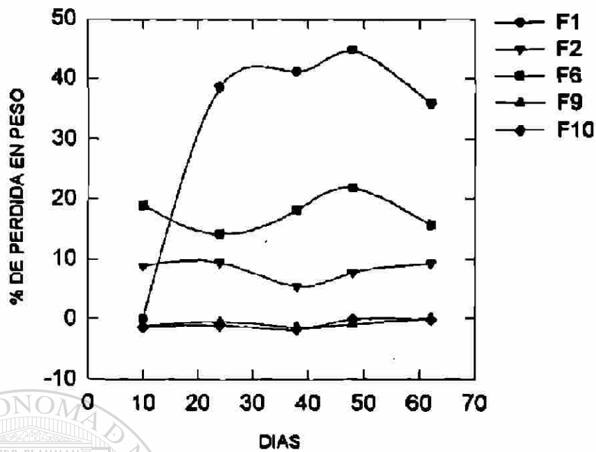
Fig. 13 Porcentaje de pérdida en peso en membranas del grupo 1 después de 62 días de exposición en río.
