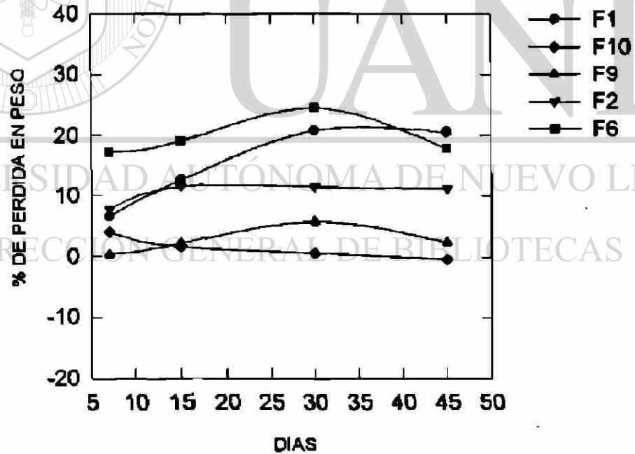
Fig. 2 Porcentaje de pérdida en peso en membranas del grupo 1 expuestas al consorcio LD-76 en laboratorio por 45 días.
