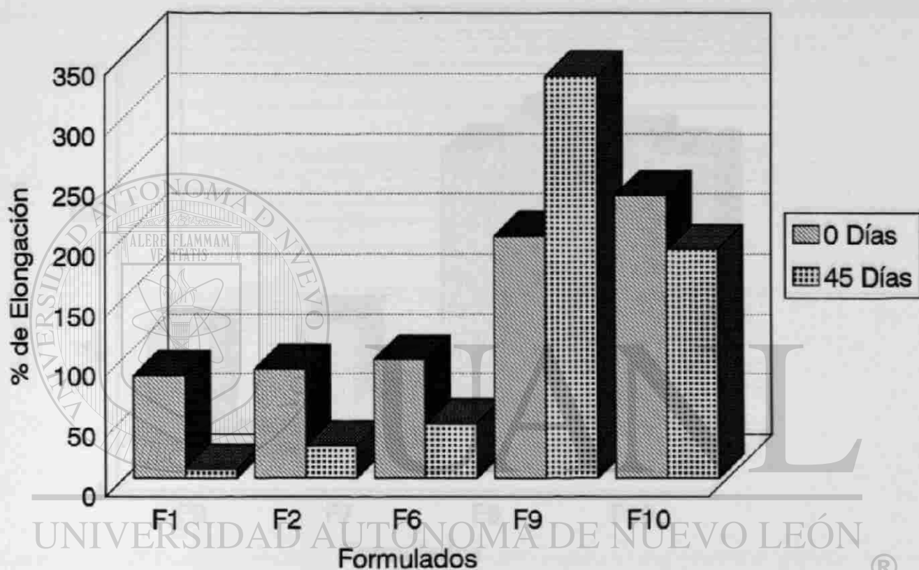
Fig.15 Porcentaje de Elongación de Formulados del Grupo 1(Almidón), después de 45 días de exposición al consorcio bacteriano LD-76.
