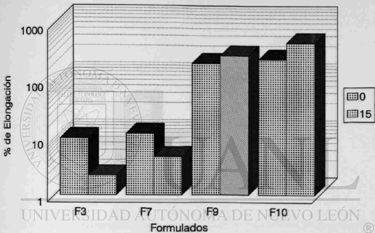
Fig. 28 Porcentaje de Elongación de los Formulados del Grupo 2 (Quitina), después de 15 días de exposición en suelo. Octubre'94-Enero'95.
