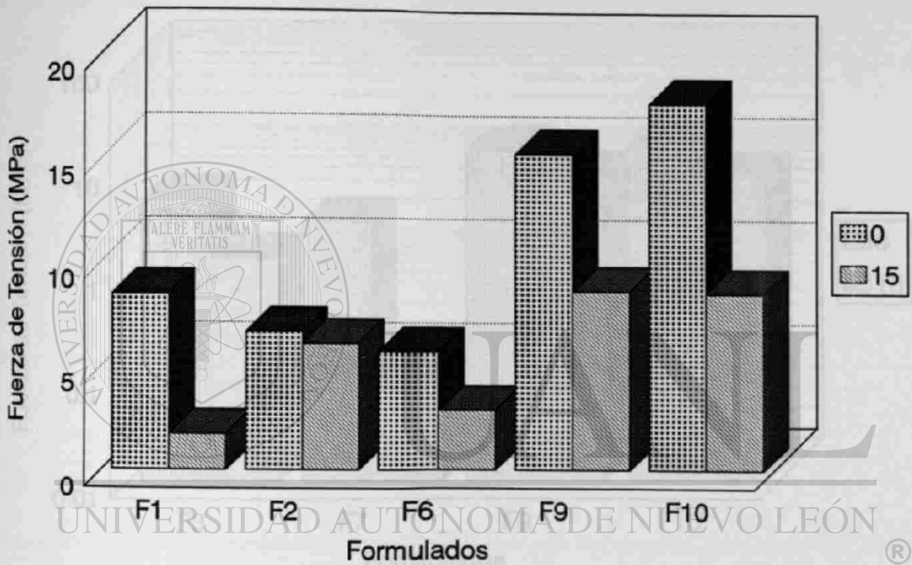
Fig. 30 Fuerza de Tensión de los Formulados del Grupo 1(Almidón), después de 15 días de exposición en suelo. Octubre'94-Enero'95.
