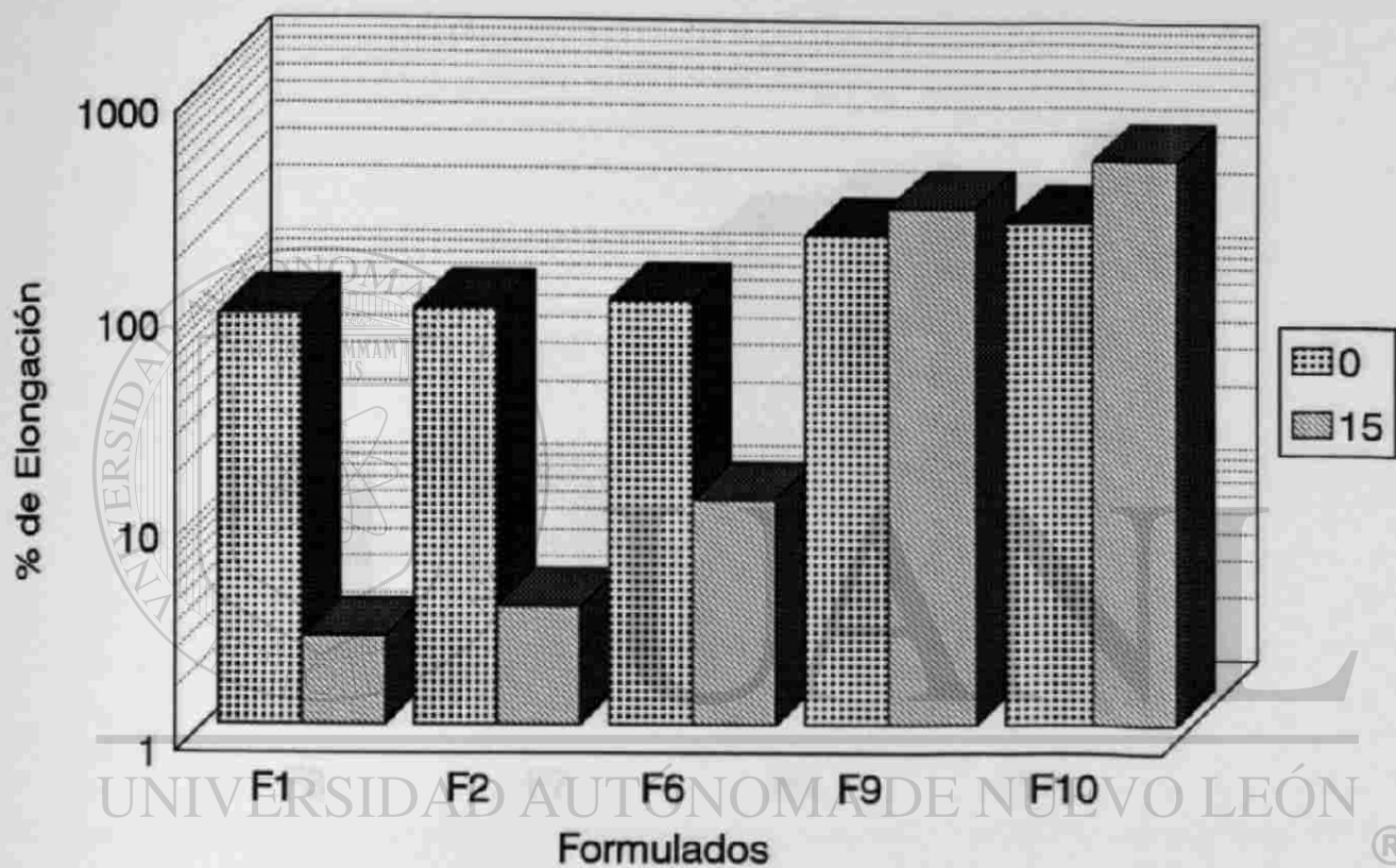
Fig. 27 Porcentaje de Elongación en Formulados del Grupo 1 (Almidón), después de 15 días de exposición en suelo. Octubre'94-Enero'95.
