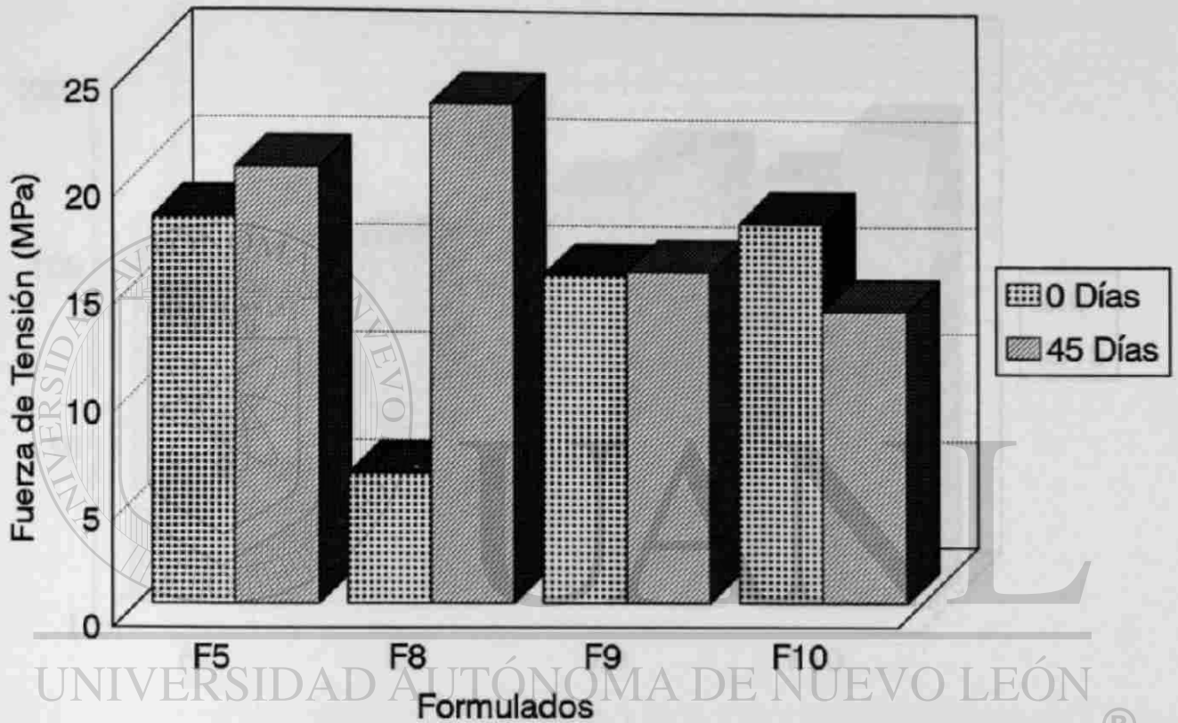
Fig.20 Fuerza de Tensión de Formulados del Grupo 4 (Pectina), después de 45 días de exposición al consorcio bacteriano LD-76.
