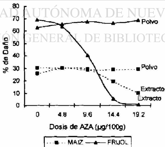
FIGURA 4. Daño al grano de maíz y frijol tratado con polvo y extracto de hoja de nim.
