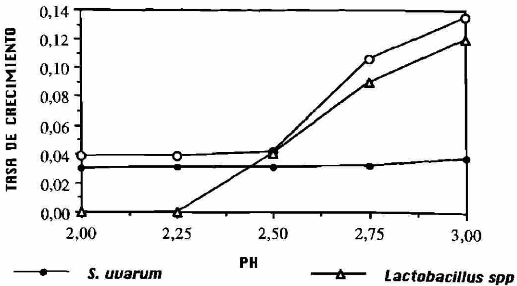
Figura No 23 Efecto del pH sobre la tasa de crecimiento de los microorganismos ( 16.0 \times 10^6 cel. / ml ), a 150 min. de exposición.
