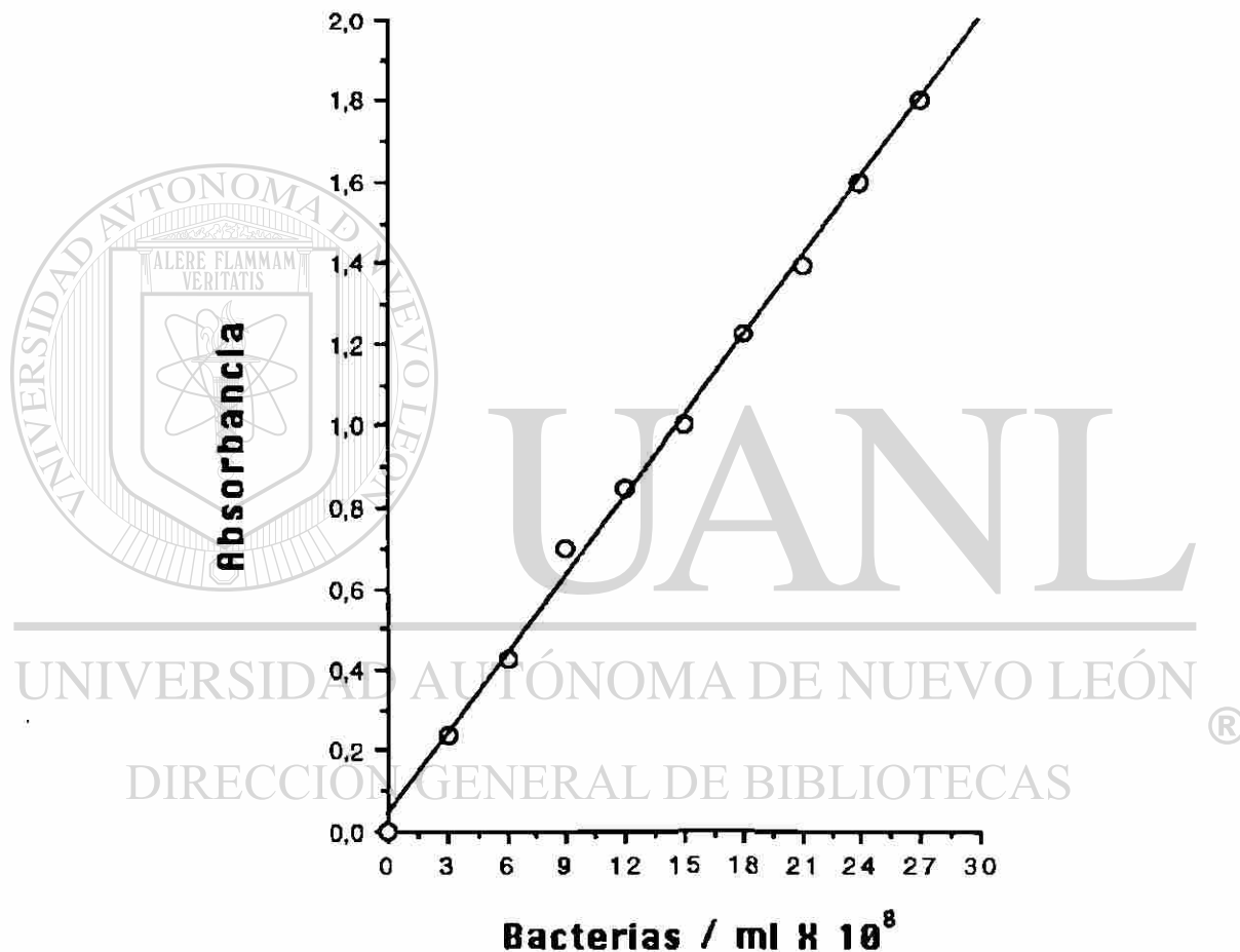
Figura No 1 Curva de calibración para determinar turbidez o el número de microorganismos/ml para Pediococcus spp y Lactobacillus spp .
