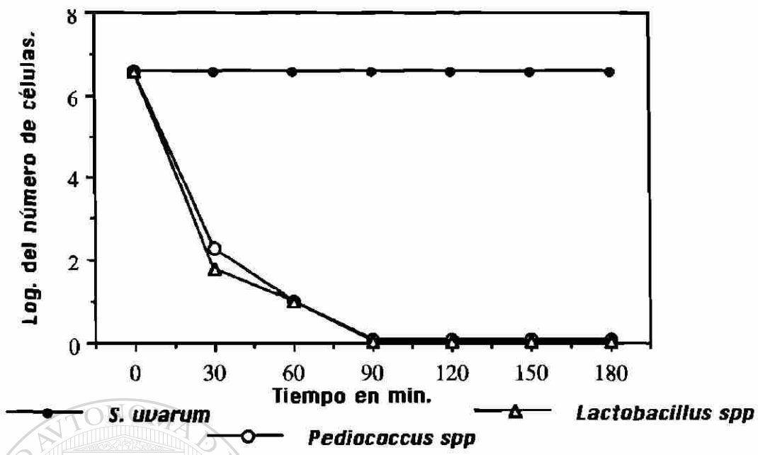
Figura No 37 Efecto bactericida del pH de 2.75 sobre los microorganismos a una concentración de 4.0 \times 10^6 células por ml.
