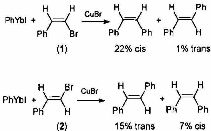
Figura 33. Reacción de acoplamiento de PhYbl con cis y trans-Bromuro de Estirilo.
