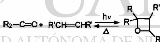
Figura 2. Obtención de oxetano
