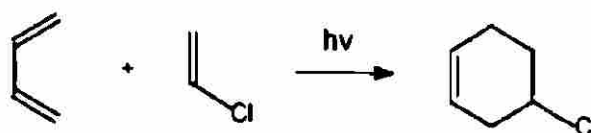
Figura 3. Reacción Diels-Alder
