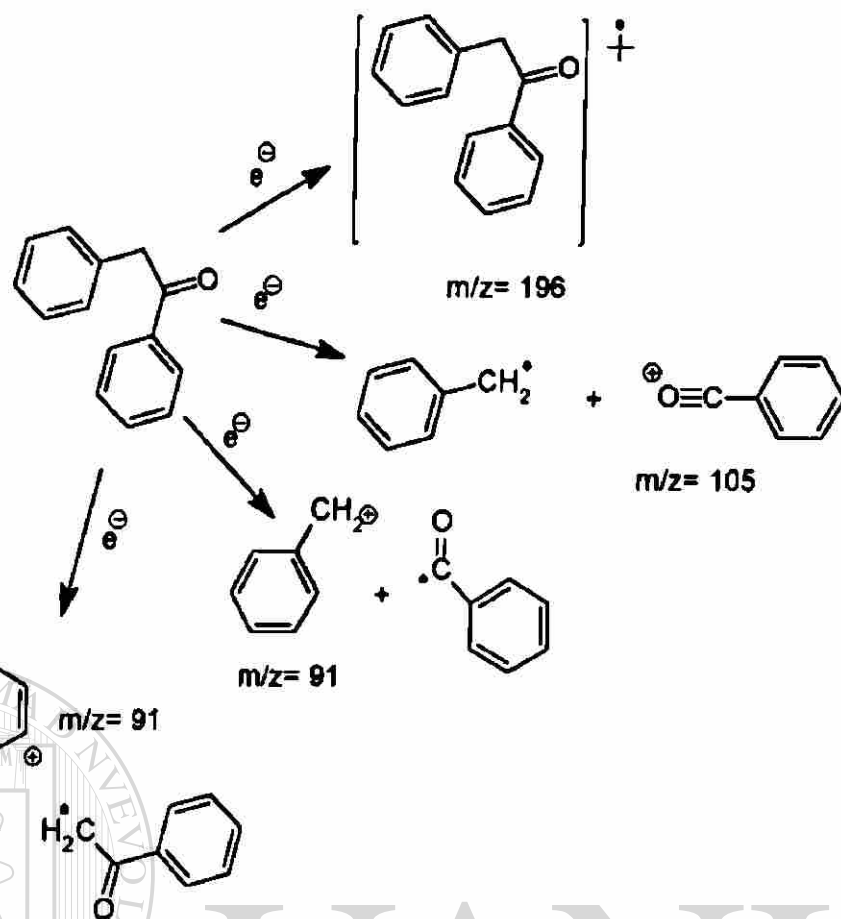
Figura 61. Componentes detectados por masas, de la reacción de la sal bromuro de tributilbencilfosfonio con 1-fenil-1-trimetilsililmetanona.
