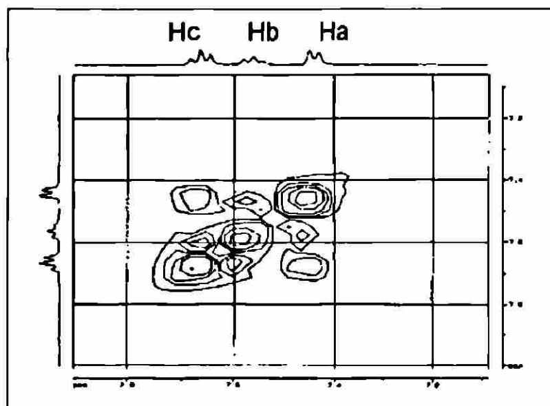
Figura 69. Espectro de COSY del 1,2-difenil,1,2-bis(trimetilsilieteno).
