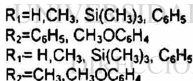
Figura 38. Ruta sintética para la obtención de derivados de estilbeno empleando la metodología de Corey.
