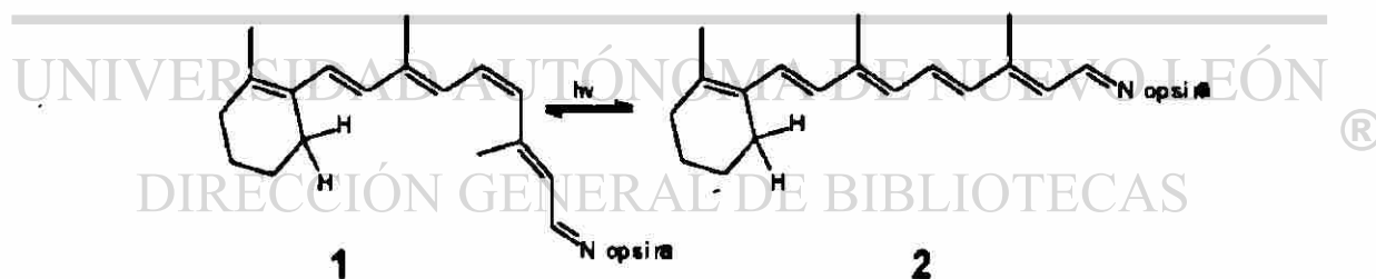
Figura 16. Ejemplo de sistema fotocromático basado en la isomería cis-trans
