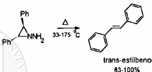
Figura 27. Obtención de cis y trans-estilbeno por descomposición térmica.
