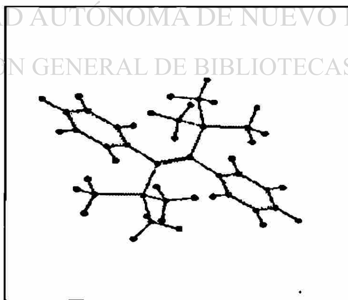
Figura 70. Estructura modelada del 1,2-difenil,1,2bis(trimetilsilieteno).
