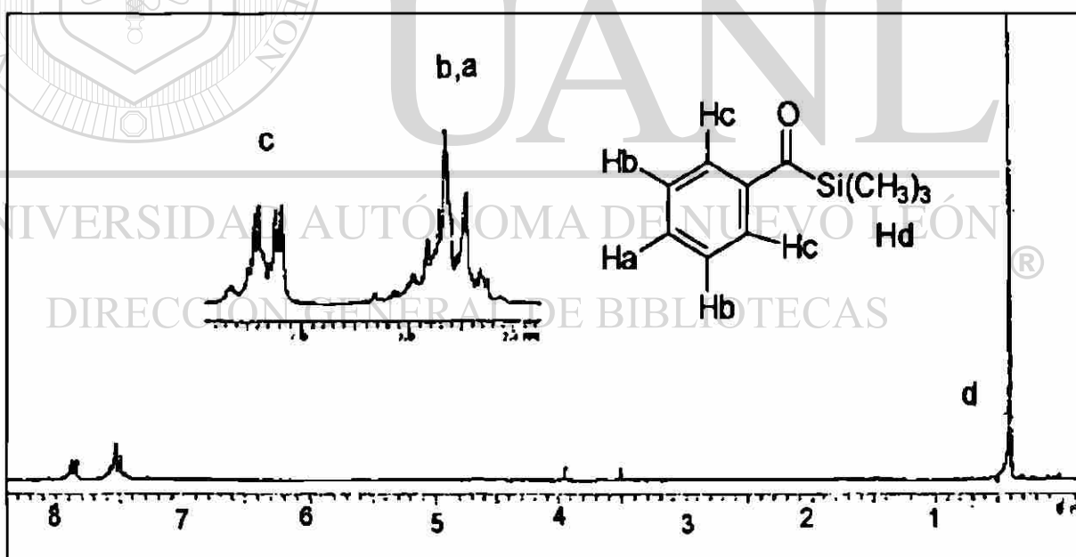
Figura 54. Espectro de ^1\text{H} RMN de 1-Fenil-1-trimetilsililmetanona.
