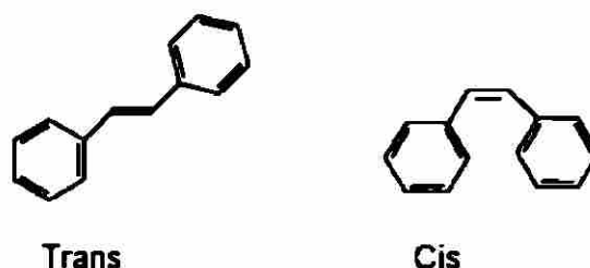
Figura 20. Isómeros de estilbeno.
