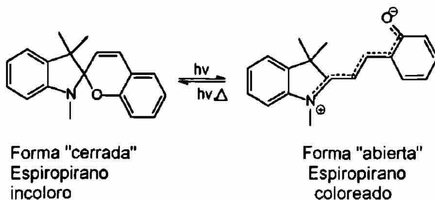
Figura 12. Interconversión fotocromática de espiropiranos
