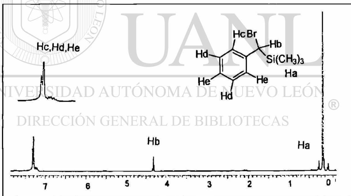
Figura 46 . Espectro de ^1H RMN de bromofeniltrimetilsililmetano.
