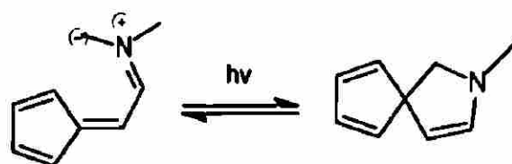
Figura 11. Reacción electrocíclica 1,5.
