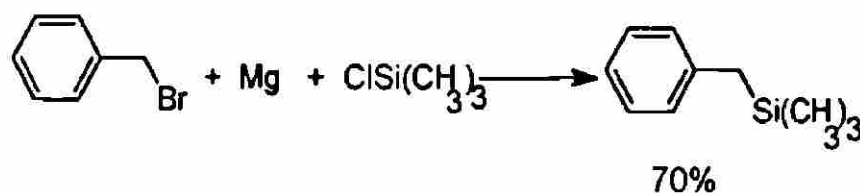
Figura 45. Reacción del bromuro de bencilmagnesio con clorotrimetilsilano.
