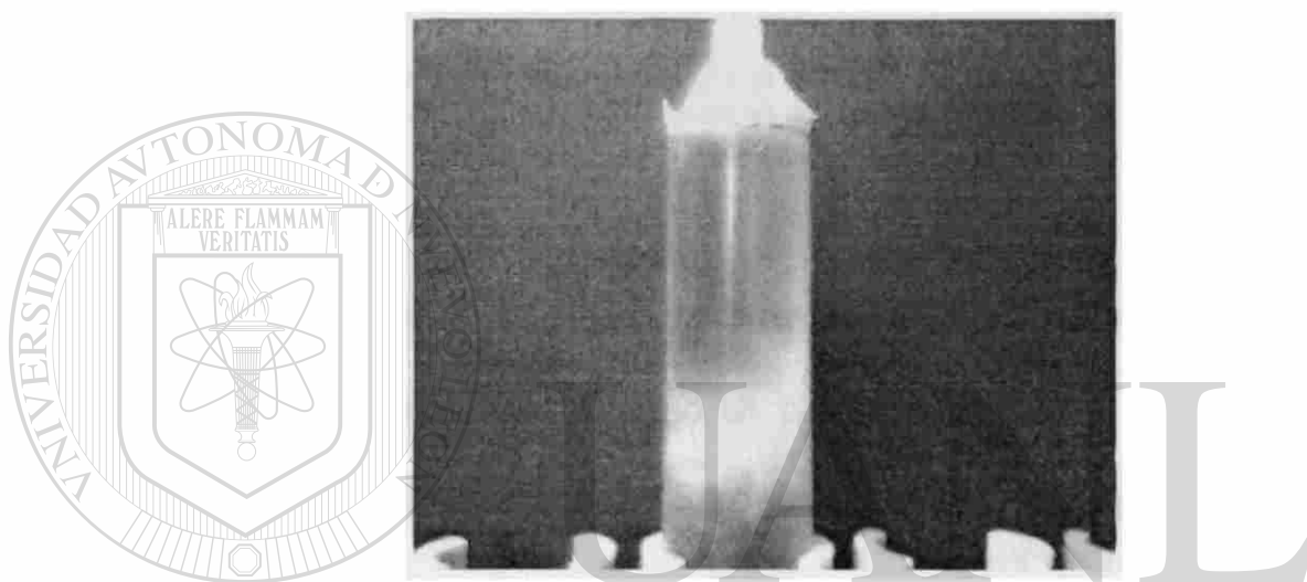
Figura 3. Purificación de las partículas fágicas. Las partículas fágicas se separaron por centrifugación en un gradiente de CsCl. La banda blanca corresponde a los fagos.
