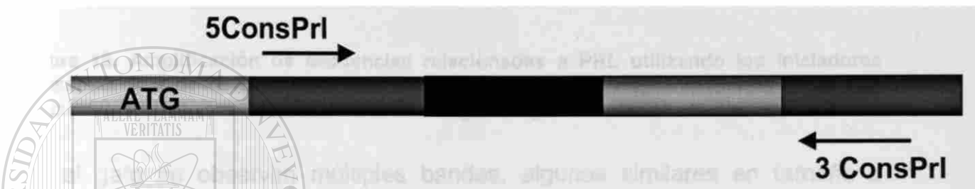
Figura 17. Iniciadores consenso. Se esquematizan los sitios de unión de los iniciadores consenso sobre los DNACs de la familia de la PRL.
