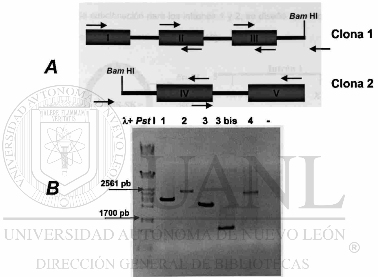
Figura 11. Análisis de los intrones. (A) Esquema donde se representa la estructura de las dos clonas obtenidas a partir del PA de PRL. Se indican los sitios de unión de los iniciadores. (B) Gel de agarosa al 0.8 % donde se resolvieron los productos amplificados de los intrones. Los carriles están numerados de acuerdo al PA del intrón correspondiente. Para el intrón 3 se muestran dos carriles el primero corresponde al PA desde el exón III hasta el sitio Bam HI mientras que el segundo corresponde al PA que inicia en el sitio Bam HI y termina en el exón IV. Se incluyó un testigo negativo de PCR (-).
