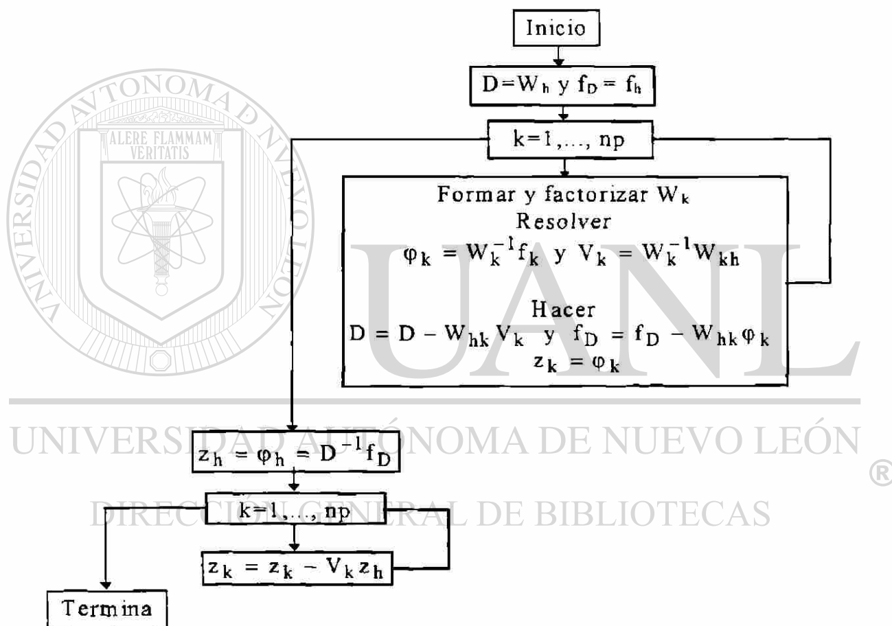
Fig. 3.3 Algoritmo para la solución eficiente de Wz=f(z) .
