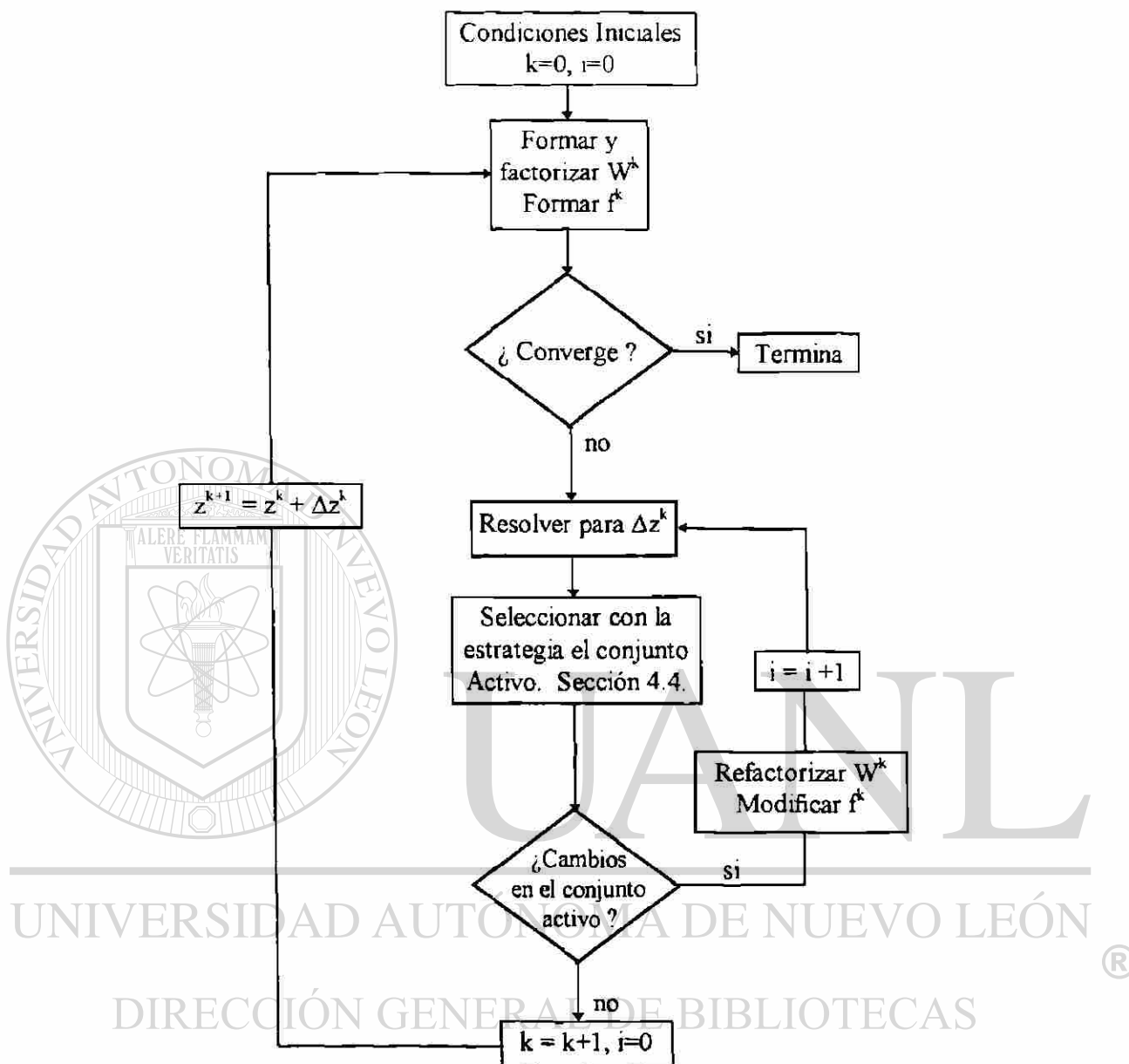
Fig. 4.2 Algoritmo general para la solución de la coordinación hidrotérmica
