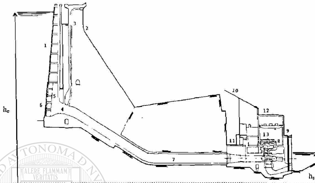
Fig. 2.4 Planta hidroeléctrica de almacenamiento.
