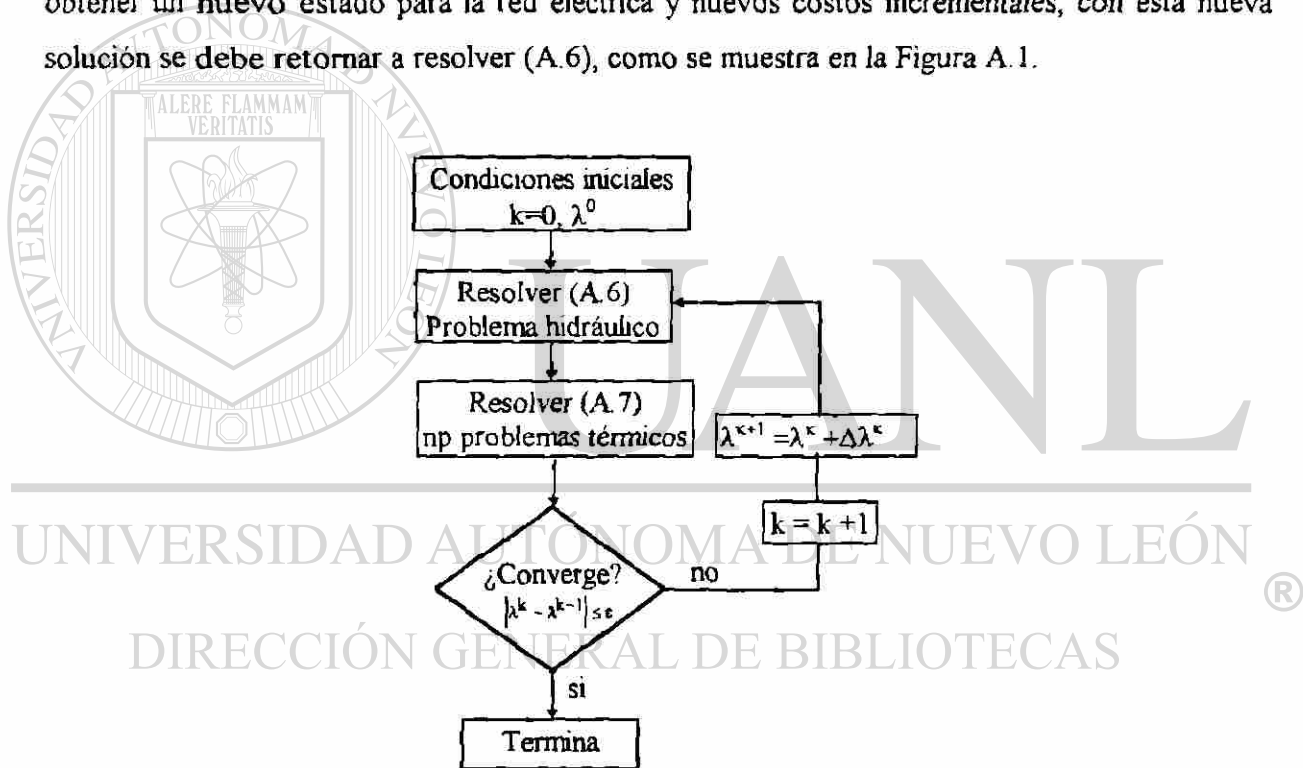
Fig. A.1 Diagrama de bloques para algoritmo de descomposición
