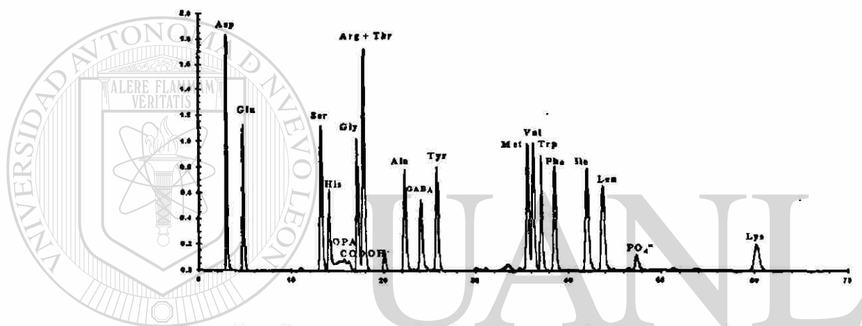
Figura 17. Cromatograma obtenido de una mezcla de estándares de AAs de 4.17 nmol/ml empleada para determinar las condiciones de trabajo óptimas en el CLAR.
