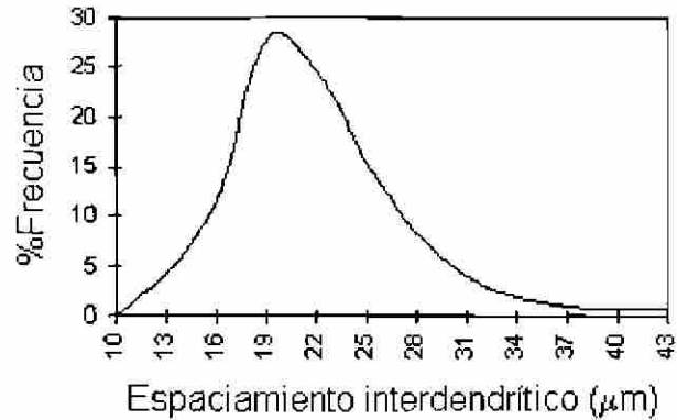
Fig. 5.19. Curva de frecuencias de los espaciamientos interdendríticos.
