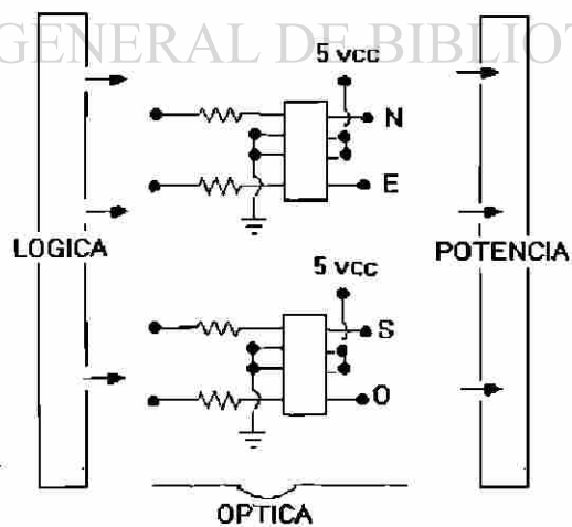
Figura 4.5: Sección Óptica.
