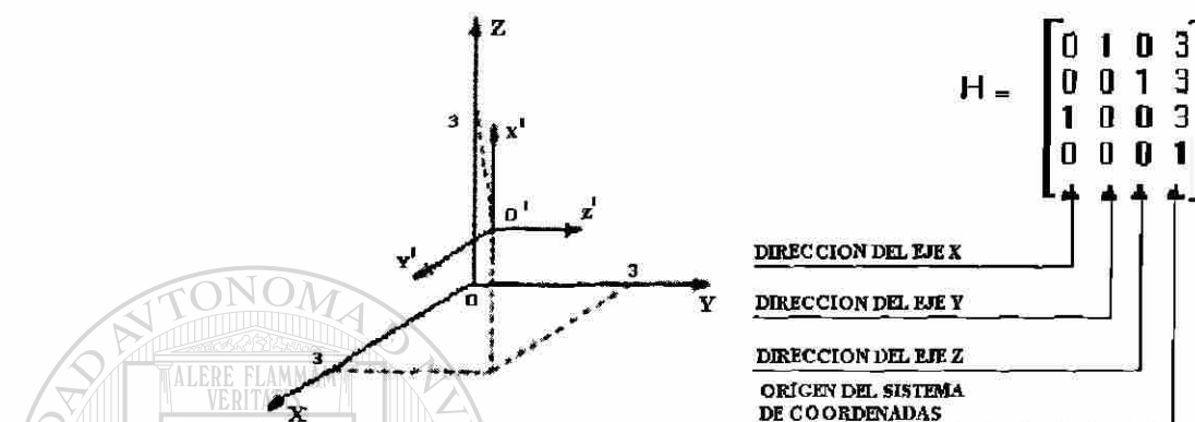
Figura 5.2: Obtención del sistema de referencia definido por la matriz transformada H .
