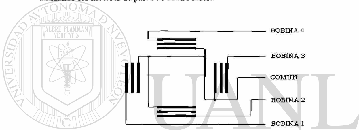
Figura 4.2: Motor de pasos de 4 fases.
