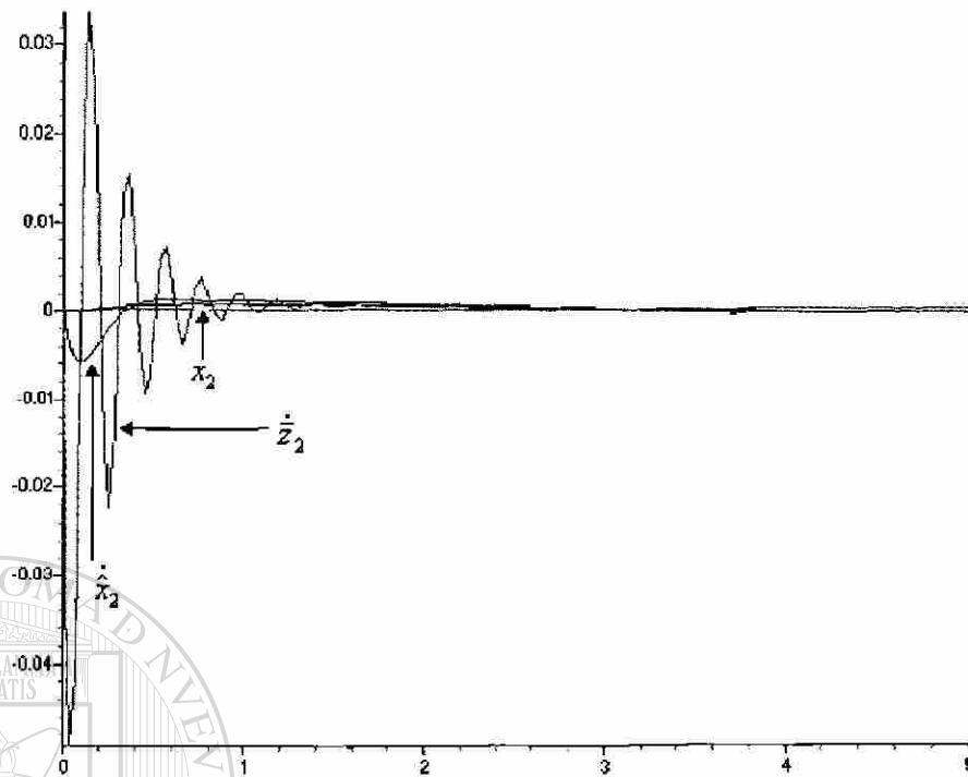
Figura 3.3: El estado x_2 con los estimados \hat{z}_2 y \hat{x}_2 .
