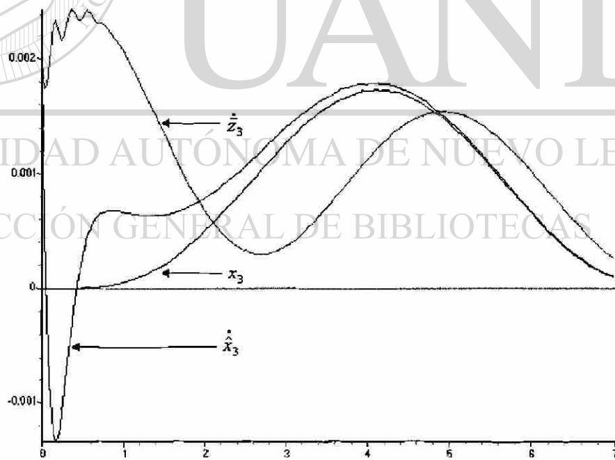
Figura 3.4: El estado x_3 con los estimados \hat{z}_3 y \hat{x}_3 .
