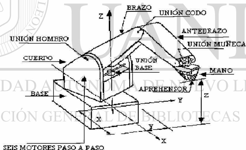
Figura 4.1: Robot TIGRE 01 .
