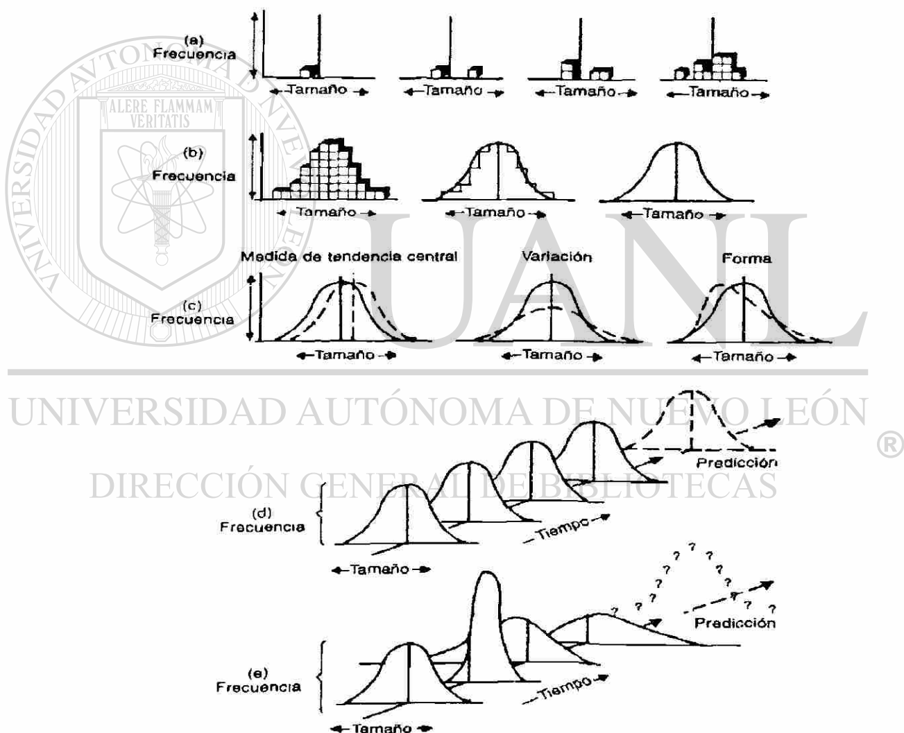
Figura 2.(1,2,3) Variaciones Naturales
