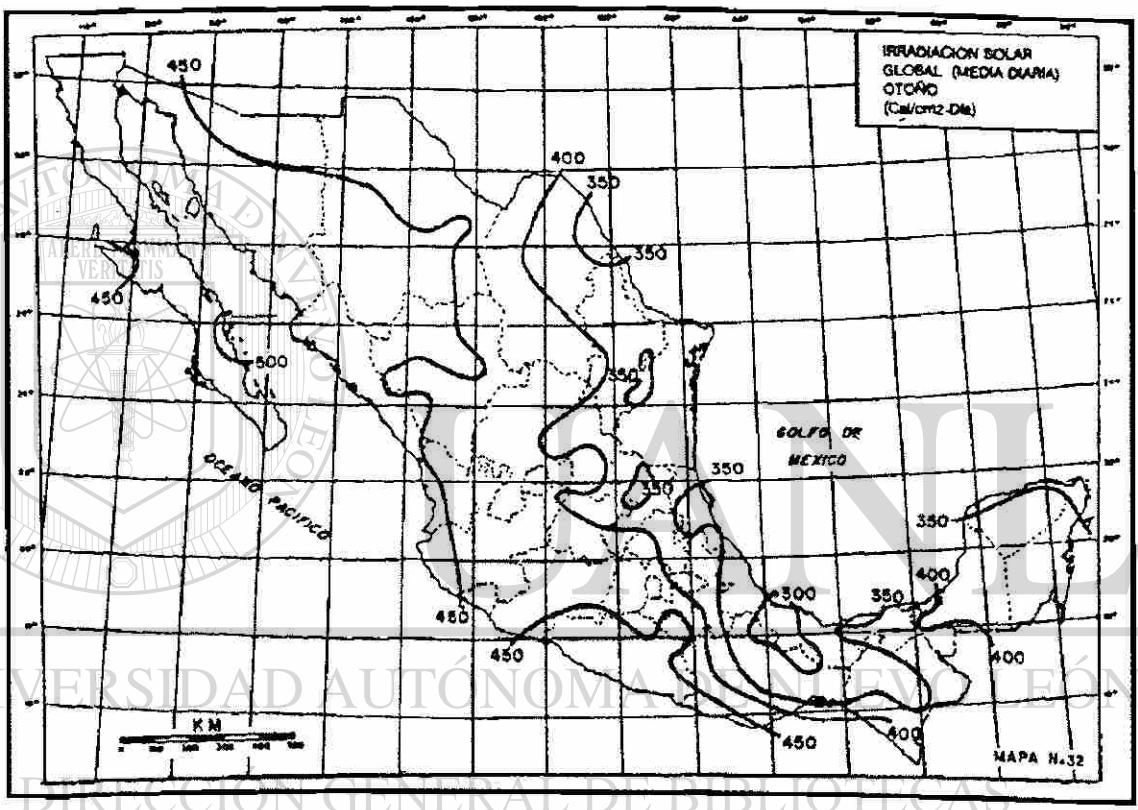
Figura 3. Mapa de insolación global en otoño
