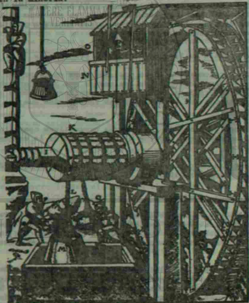
Rueda de arcaduccs para extraer el agua de las minas. Agricola, 1556.
